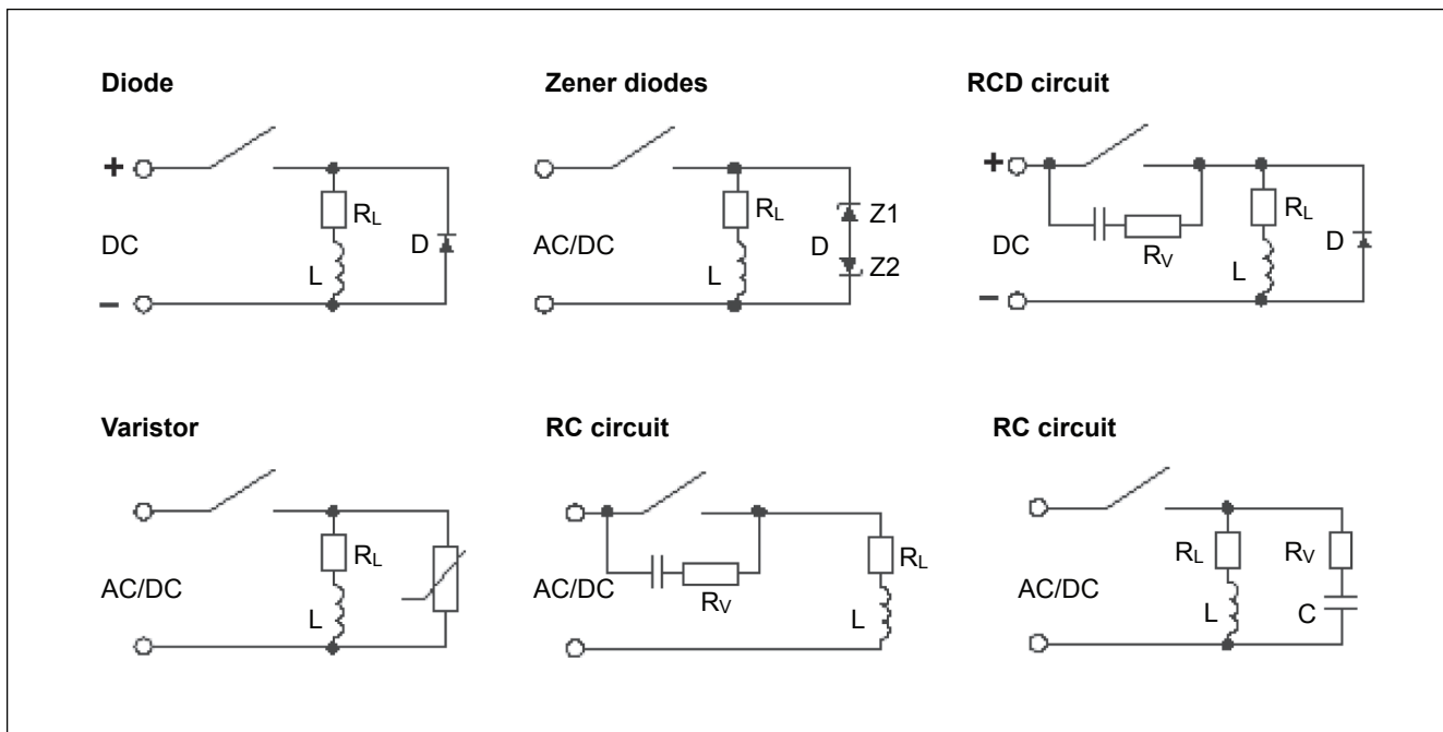
Fig. 23. Protection circuits
